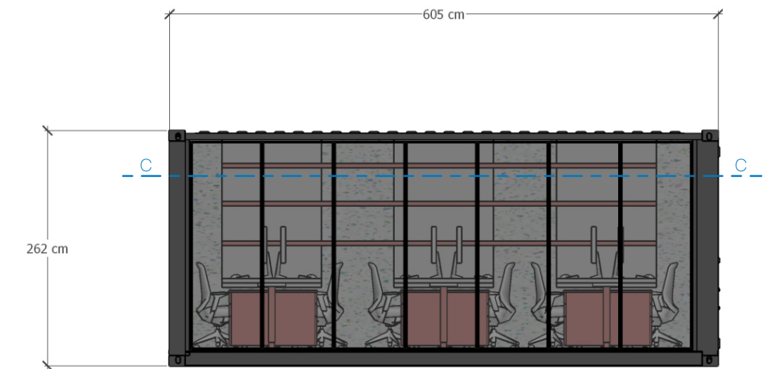
V.FRONTALE
