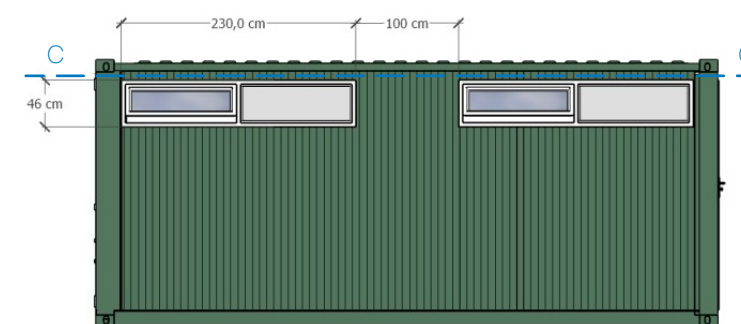
FRONTALE
