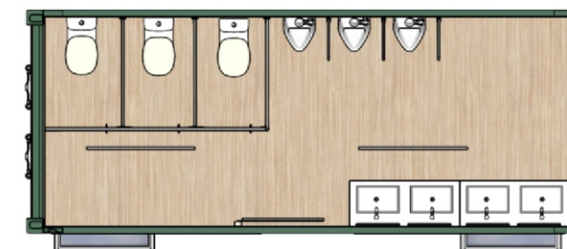
SEZIONE C-C
