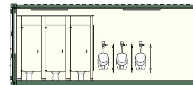
SEZIONE B-B
